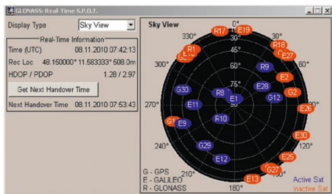
Рисунок 2. Гибридная спутниковая группировка, отображающая спутники ГЛОНАСС (R), GPS (G) и Galileo (E)
