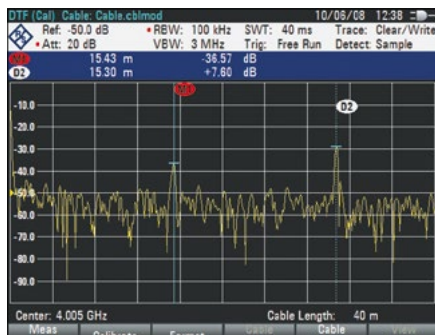
Измерение расстояния до места повреждения (DTF)
