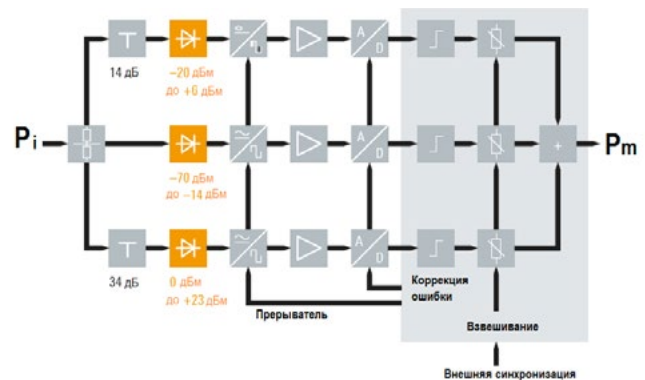
Архитектура 3-канального датчика
