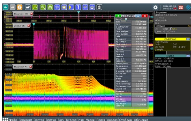
Пример анализа импульсного сигнала
