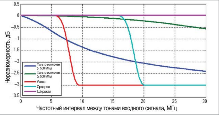
Рисунок 2. Неравномерность измерения отношения пиковой мощности к средней для измерителей U2021XA/22XA при двухтональном входном сигнале (для следующих установок видеополосы: широкая, средняя, узкая и "фильтр выключен").
