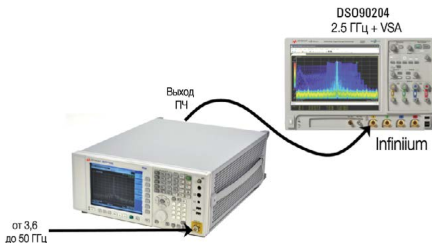
Рисунок 3. Анализатор сигналов Keysight PXA используется в качестве широкополосного понижающего преобразователя частот. Для дискретизации широкополосной ПЧ (до 900 МГц) используется внешний прибор, например, осциллограф. Обработка сигнала для анализа спектра, демодуляции и векторных измерений выполняется с помощью ПО векторного анализа сигналов Keysight 89600 VSA, работающем на осциллографе или на ПК.
