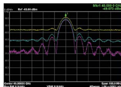
Рисунок 9. Качество измерений параметров низкоуровневого сигнала на частоте 49 ГГц значительно улучшено за счет применения малошумящего сигнального тракта и функции снижения собственных шумов анализатора Keysight PXA. Верхняя трасса соответствует обычному измерению, средняя трасса получена с малошумящим сигнальным трактом, а нижняя трасса демонстрирует эффект включения функции снижения собственных шумов.
