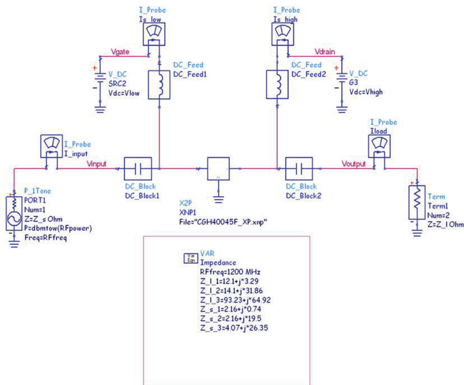
Рисунок 4 — САПР ADS упрощает создание моделей на схемном уровне и моделей X-параметров и позволяет проводить сравнения между результатами моделирования и измерения
