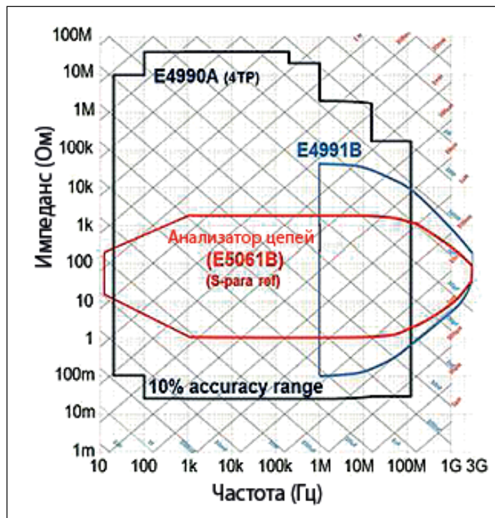
Рисунок 6. 10% степень точности измерения импеданса приборов E4990A, E4991B и E5061B
