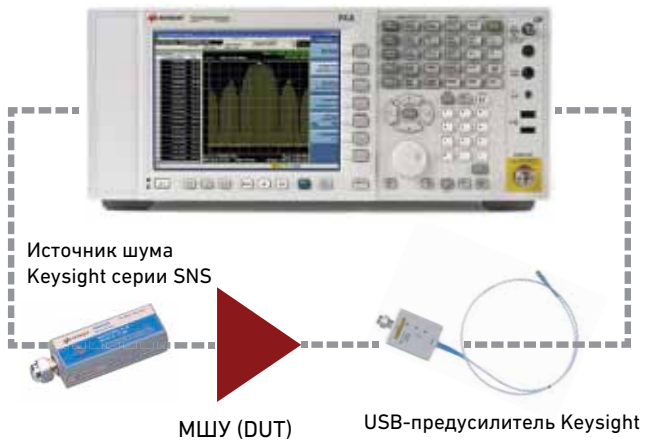
Рисунок 2. Установка, включающая предусилитель и анализатор спектра
