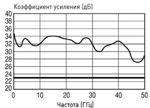
Коэффициент усиления усилителя 83051A
