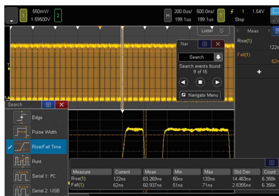
Рис. 10а. Осциллограф серии 4000 X настроен на захват сигналов с различным временем нарастания фронта. Использование функций поиска и навигации позволило найти, отметить (белые треугольники) и быстро перемещаться между шестнадцатью событиями, не соответствующими заданным критериям по времени нарастания фронтов.
