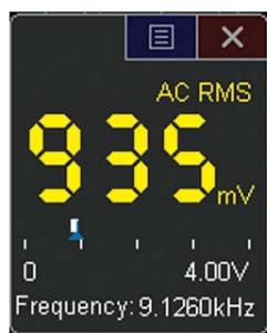
Рис. 25. Измерения с помощью 3-разрядного вольтметра и 5-разрядного частотомера будут всегда у вас под рукой.
