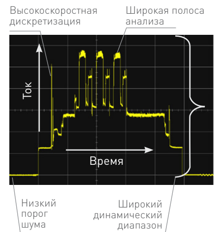
Рис. 2. Желательные ключевые требования к измерениям формы широкополосных и низкоуровневых сигналов тока.
