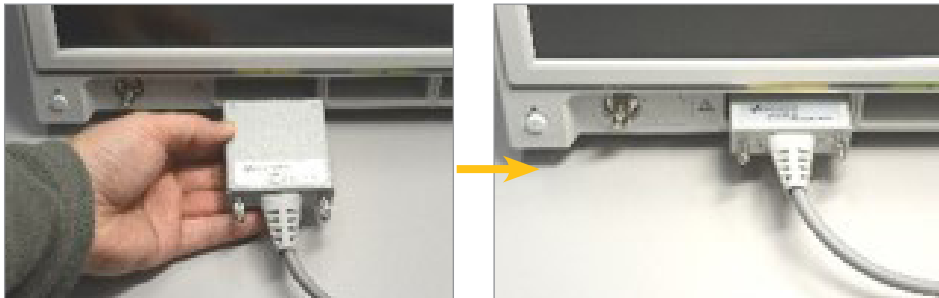
[31a] [316] Рис. 31а и 31б. Подключение датчика к каналу базового блока
