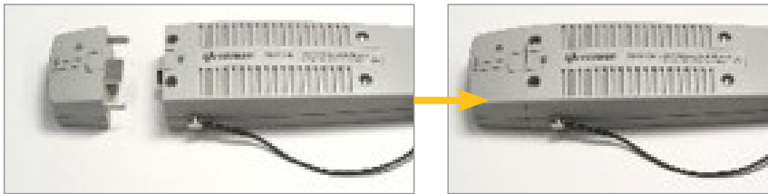
[30a] [306] Рис. 30а и 30б. Установка головки датчика на датчик тока
