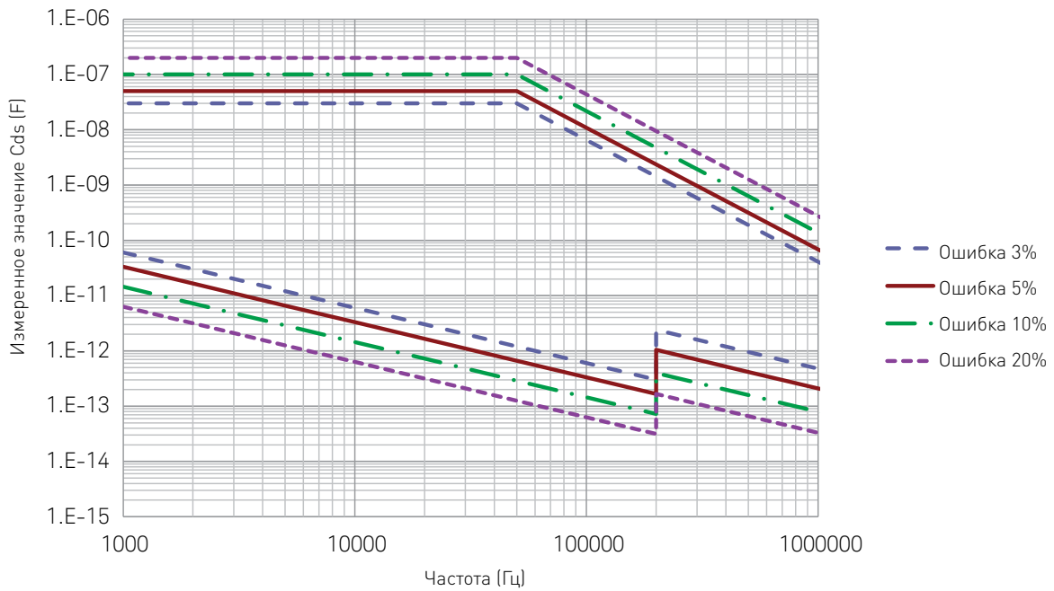
Точность измерения Cds для устройства с 3 выводами Cgs:Cds:Cgd = 1:0.1:0.01
