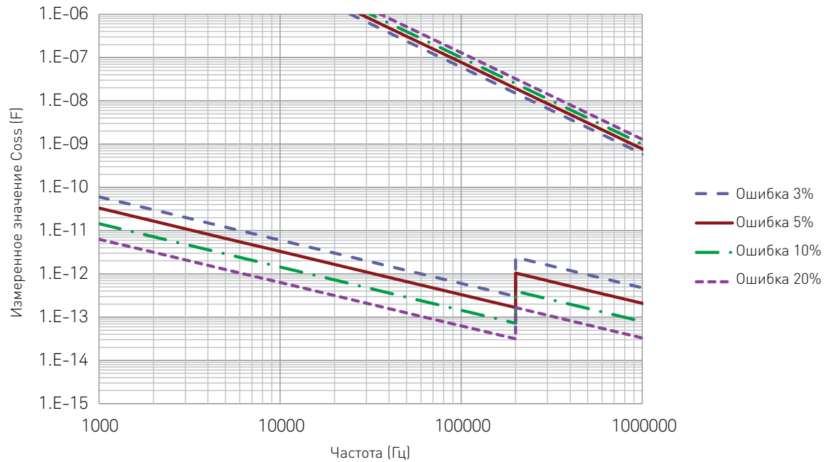
Точность измерения C_{oss} для устройства с 3 выводами C_{gs}:C_{ds}:C_{gd} = 1:0.1:0.01
